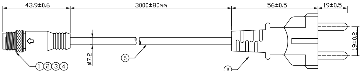
ST302歐規
